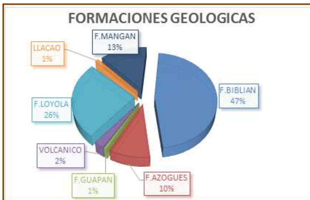
GRÁFICO NRO. 5: REPRESENTACIÓN EN PORCENTAJE DE LAS FORMACIONES GEOLÓGICAS.
