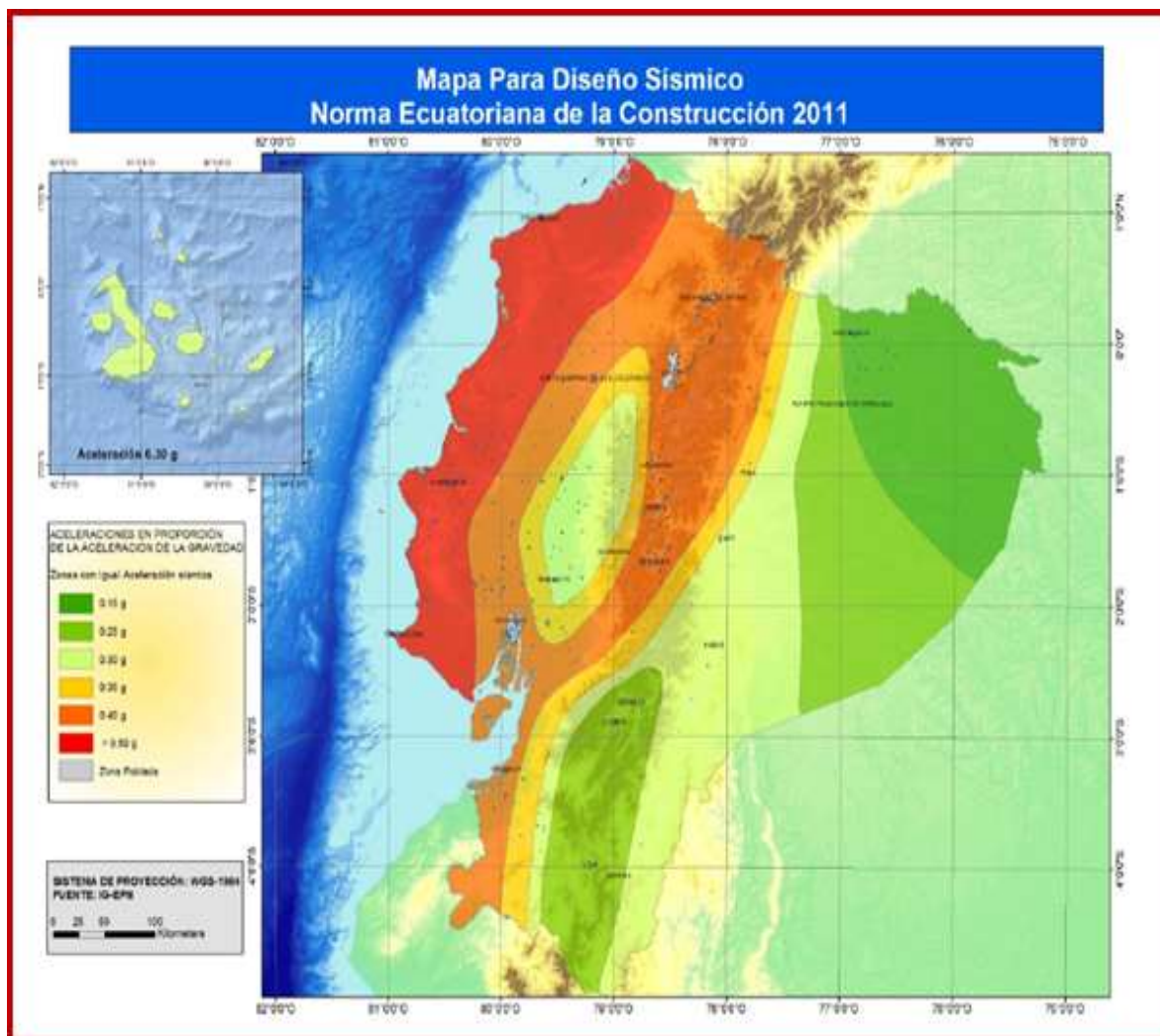
GRÁFICO NRO. 16: MAPA PARA DISEÑO SÍSMICO FUENTE: NORMA ECUATORIANA DE LA CONSTRUCCIÓN 2011 ELABORACIÓN: EQUIPO CONSULTOR
