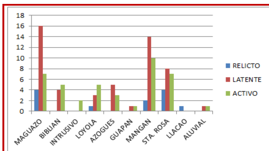
GRÁFICO NRO. 6: VULNERABILIDAD A GENERAR DESLIZAMIENTOS DE ACUERDO A LAS PROPIEDADES DE LAS FORMACIONES.
