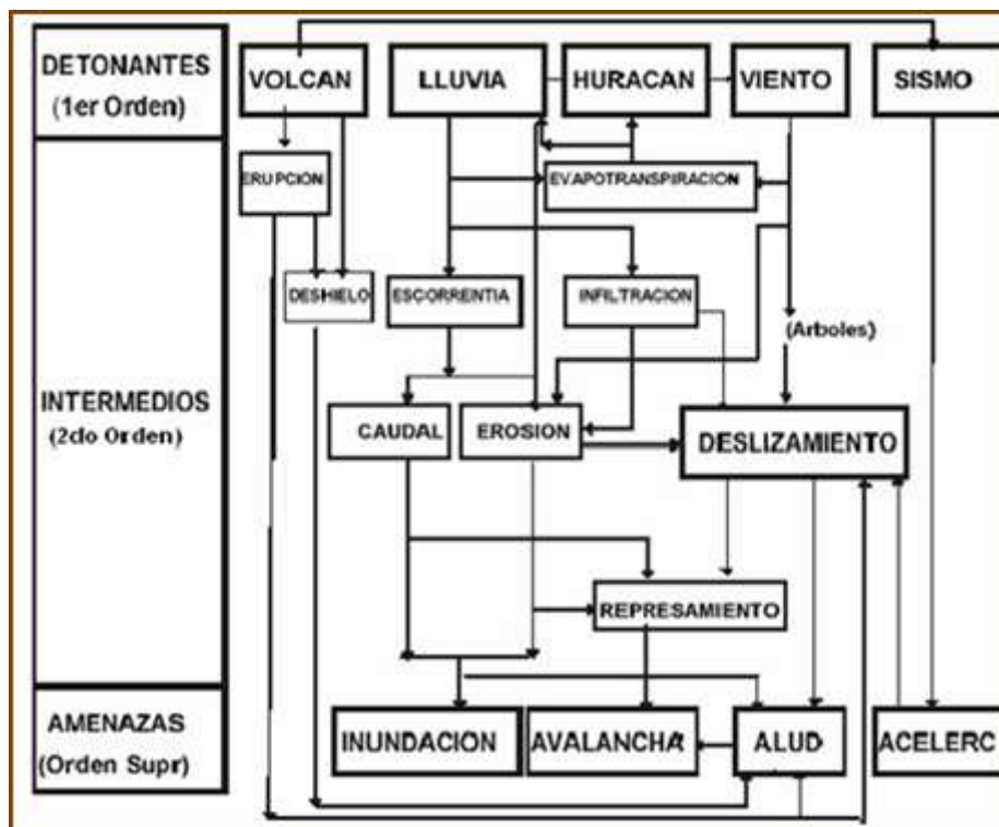
GRÁFICO NRO. 4: SECUENCIA DE EVENTOS NATURALES Y AMENAZAS FUENTE: TOMADO Y MODIFICADO DE GONZÁLEZ (2005) ELABORADO POR: EQUIPO CONSULTOR
