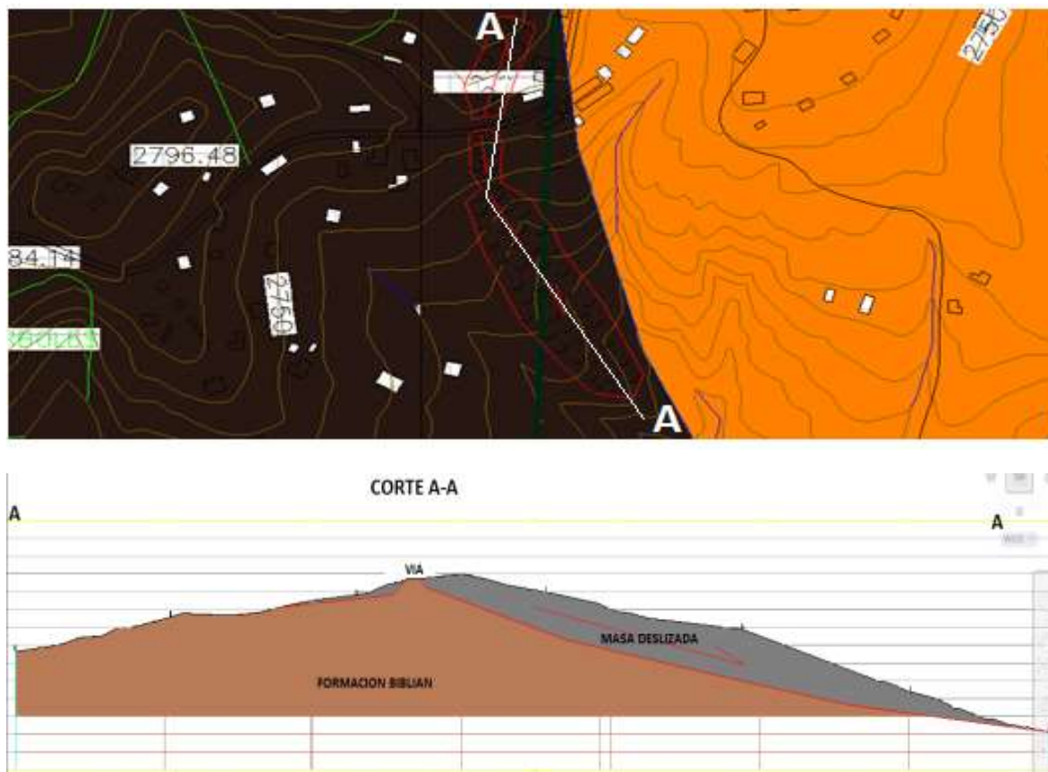
GRÁFICO NRO. 15: GEOLOGÍA DEL SECTOR FUENTE: EQUIPO CONSULTOR
